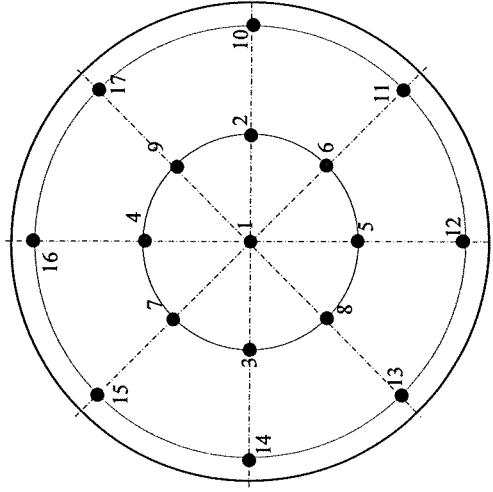
17點式
